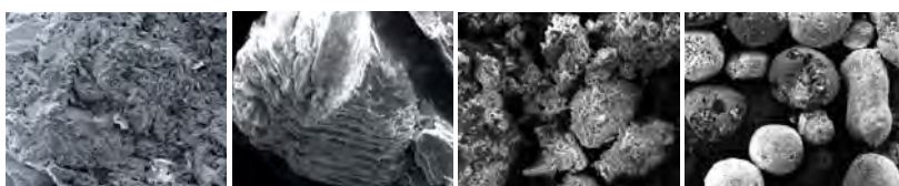
Expandierter Glimmerschiefer
